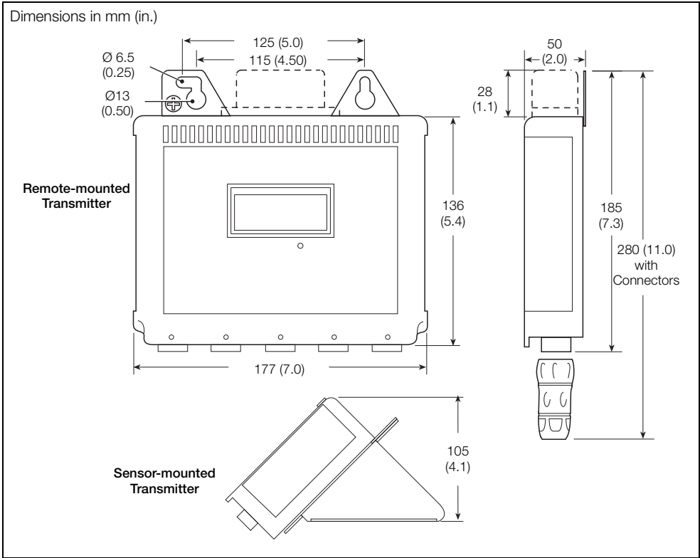
Fig. 2.19 AquaMaster 3 Dimensions
